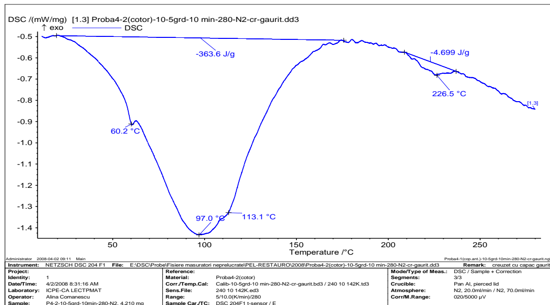
Fig. 1.10. Curba DSC pentru proba de piele P4-2
