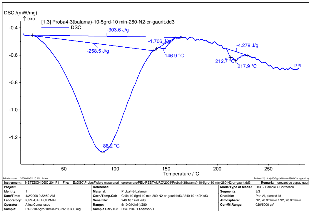
Fig. 1.11. Curba DSC pentru proba de piele P4-3
