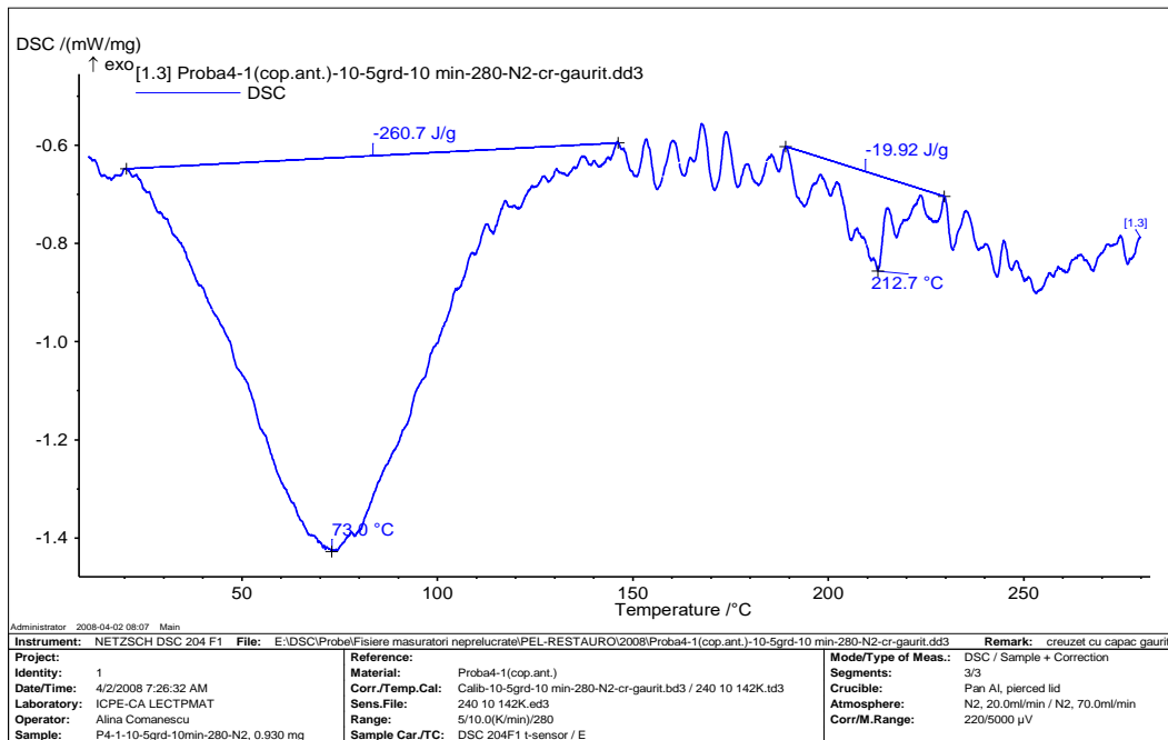
Fig. 1.9. Curba DSC pentru proba de piele P4-1
